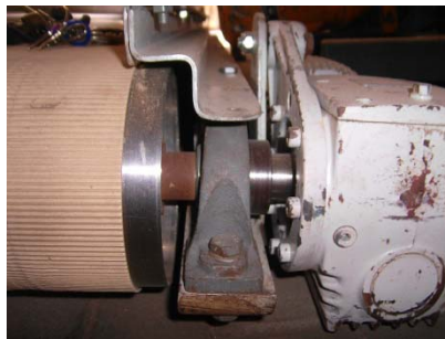
Magnetische Antriebstrommel mit Stehlager und Getriebemotor
